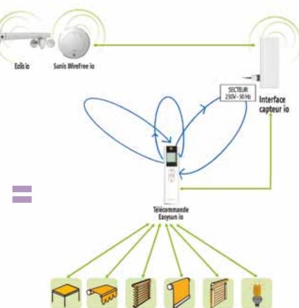
Interface capteur + Eolis / Sunis
